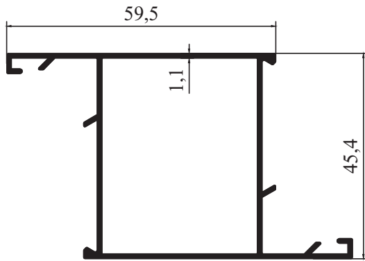
M 3005 - 0,706 kg/m
