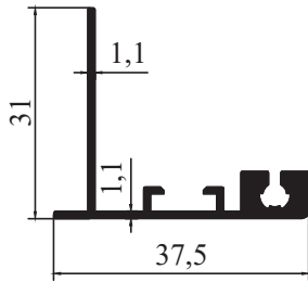
8171 - 0,353 kg/m
