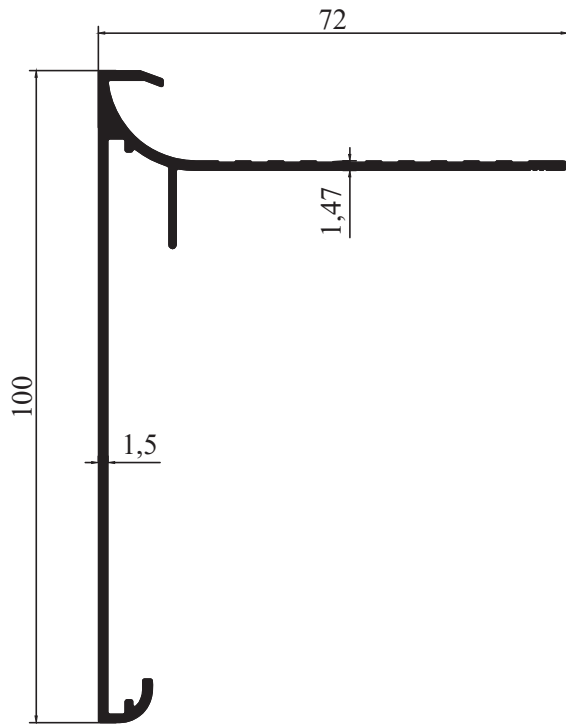
M 8548- 0,829 kg/m
