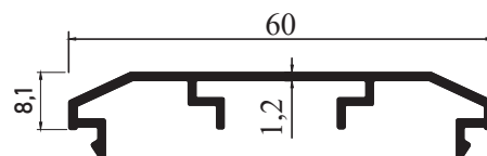
M 3108 - 0.342 kg/m
