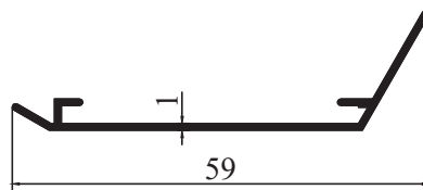
2018 - 0,220 kg/m
