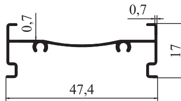
8371 - 0,206 kg/m
