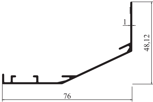
1134 - 0,400 kg/m
