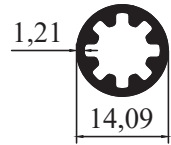
8012 - 0,203 kg/m
