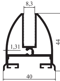
8194 - 0,837 kg/m
