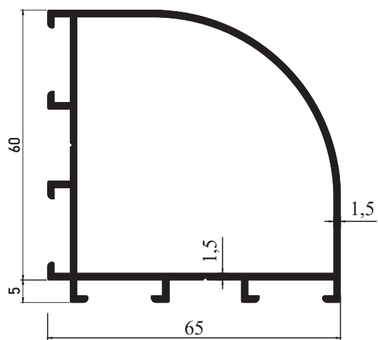
M 3106 - 1.168 kg/m
