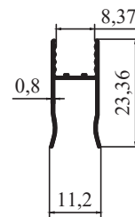
M 934 - 0,129 kg/m
