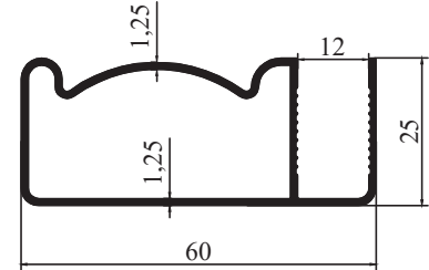
M 2075 - 0,603 kg/m
