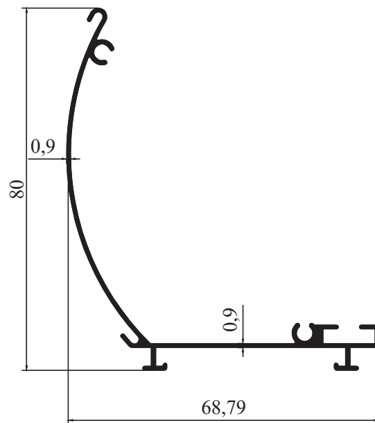
8458 - 0,502 kg/m
