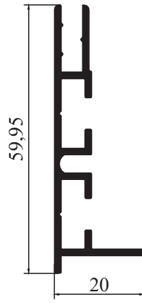
9045 - 0,530 kg/m
