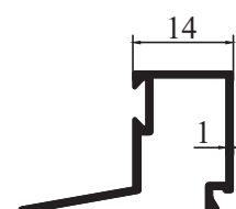
M 3021 - 0.204 kg/m
