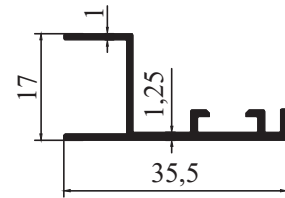
8170 - 0,228 kg/m
