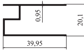
4118 - 0,273 kg/m
