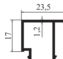
M 3111 - 0.233 kg/m
