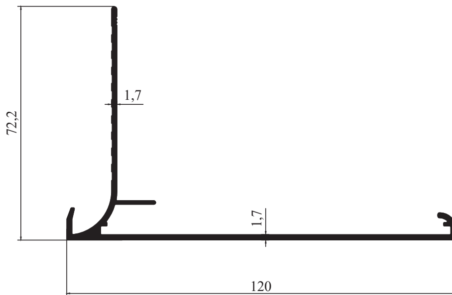
M 8549 - 1,017 kg/m
