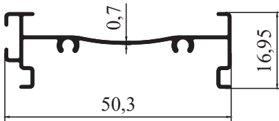
8013 - 0,234 kg/m
