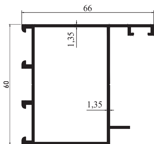
M 3105 - 1.008 kg/m
