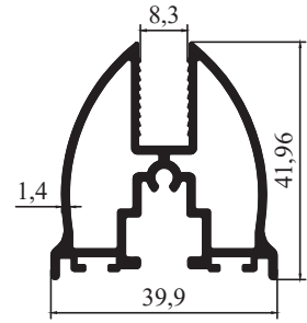
M 2114 - 0,878 kg/m
