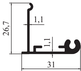
8230 - 0,290 kg/m
