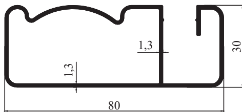
M 2076 - 0,876 kg/m
