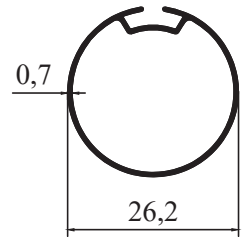
5564 - 0,171 kg/m
