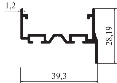
M 2155 - 0,374 kg/m
