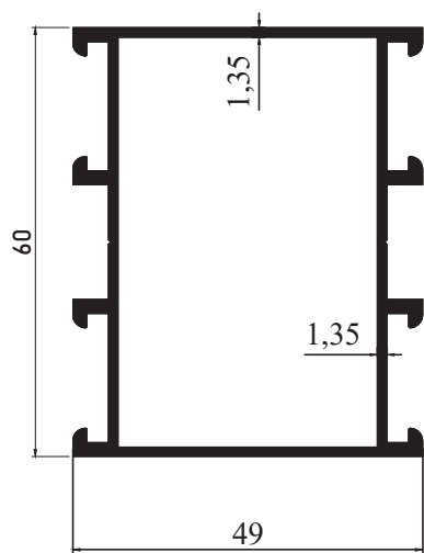
M 3101 - 0.992 kg/m
