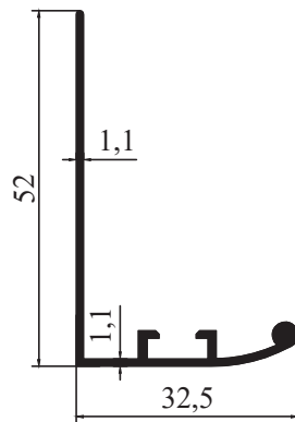
1131 - 0,312 kg/m
