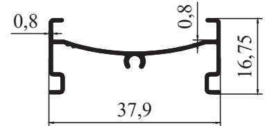
8242 - 0,198 kg/m
