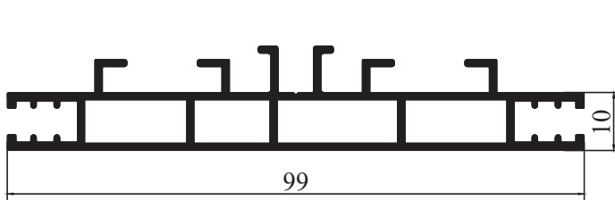
9020 - 1,109 kg/m
