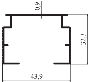
8437 - 0,347 kg/m
