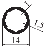
8243 - 0,144 kg/m
