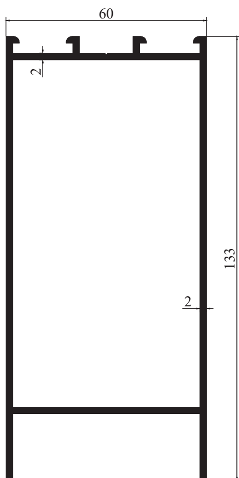
M 3109 - 2.138 kg/m
