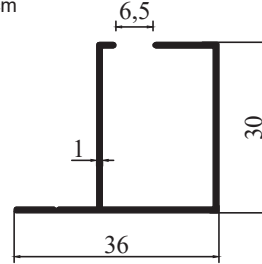
4144 - 0,289 kg/m
