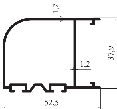
M 2156 - 0,648 kg/m
