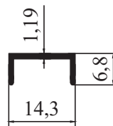
M 1528 - 0,341 kg/m
