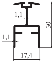
8541 - 0,272 kg/m
