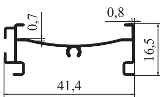
8269 - 0,206 kg/m
