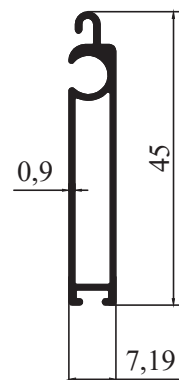
8428 - 0,277 kg/m
