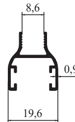
9223 - 0,205 kg/m
