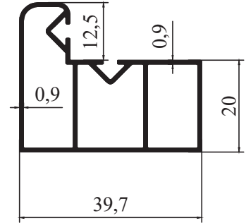
8195 - 0,469 kg/m
