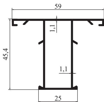
M 3003 - 0,589kg/m
