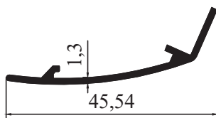
2651 - 0,222 kg/m
