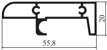
4119 - 0,544 kg/m
