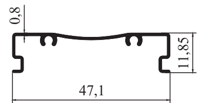
8392 - 0,207 kg/m
