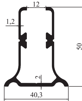
M 2064 - 0,748 kg/m
