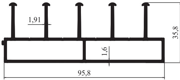
M 2202 - 1,567 kg/m
