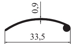
1592 - 0,108 kg/m
