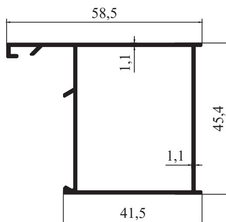
M 3004 - 0,603 kg/m
