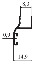
9223 - 0,140 kg/m
