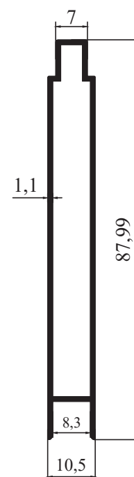
M 3023- 0,572 kg/m
