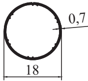
8478 - 0,107 kg/m
