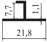
8899 - 0,104 kg/m
