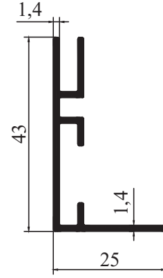
M 9201 - 0,377 kg/m
