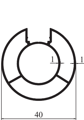
M 2011 - 0,642 kg/m
