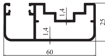
M 2071 - 0,781 kg/m
