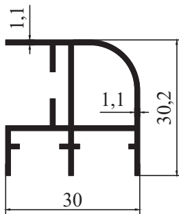
8539 - 0,418 kg/m
