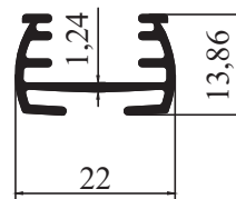
8552 - 0,224 kg/m
