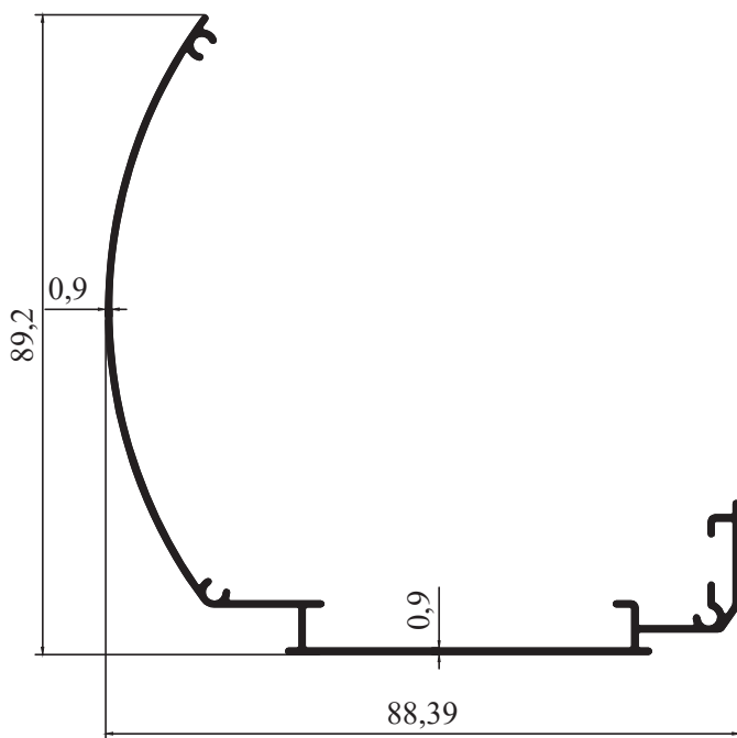
8131 - 0,543 kg/m
