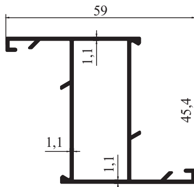
M 3002 - 0,601 kg/m
