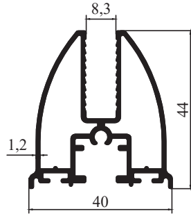
M 2112 - 0,840 kg/m
