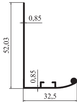
1128 - 0,241 kg/m
