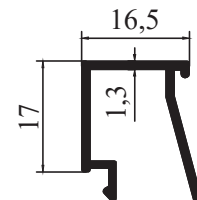
M 3112 - 0.225 kg/m
