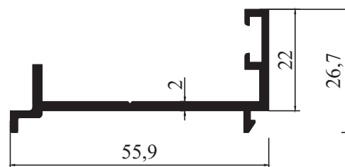
M 3107 - 0.513 kg/m
