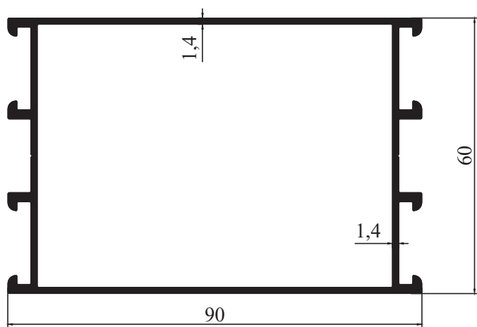
M 9514- 1,328 kg/m
