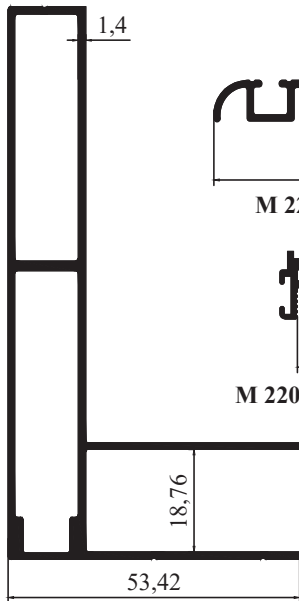
M 2210 - 1,181 kg/m
