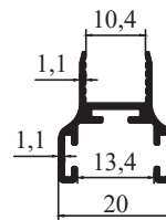
M 2135 - 0,240 kg/m
