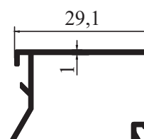
M 3020 - 0.210 kg/m
