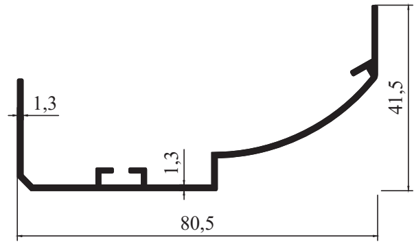
2650 - 0,526 kg/m
