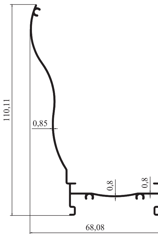
8442 - 0,561 kg/m
