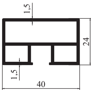
M 2055 - 0,678 kg/m
