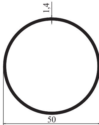
M 1500 - 0,575 kg/m
