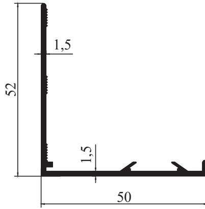
1144 - 0,464 kg/m
