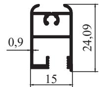
4130 - 0,254 kg/m
