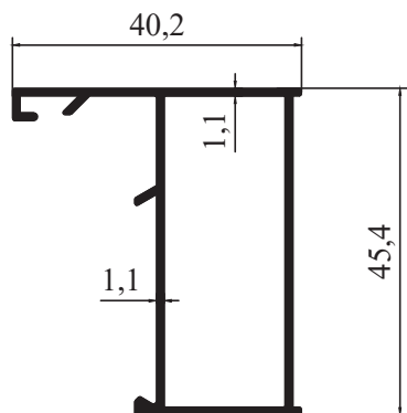
M 3001 - 0,493 kg/m
