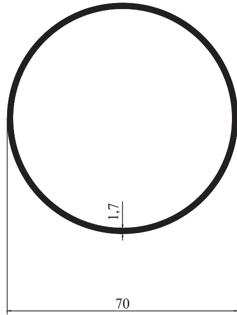
M 9524 - 0,989 kg/m
