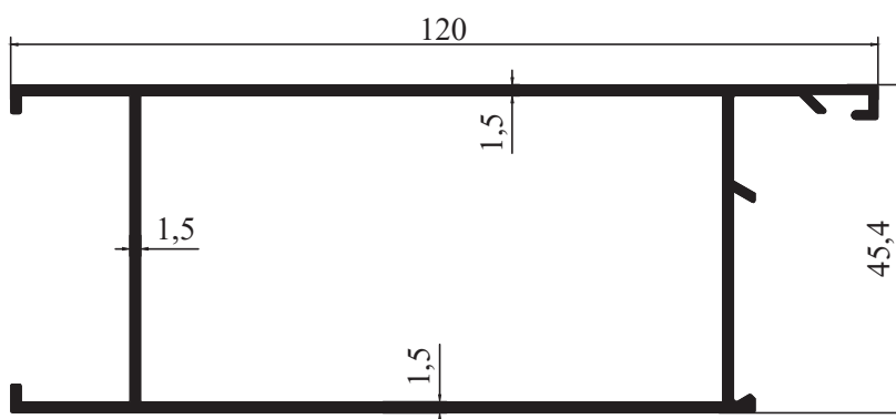
M 3010 - 1.312 kg/m
