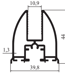
M 2113 - 0,850 kg/m
