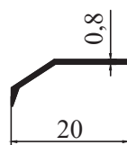
9033- 0,054 kg/m
