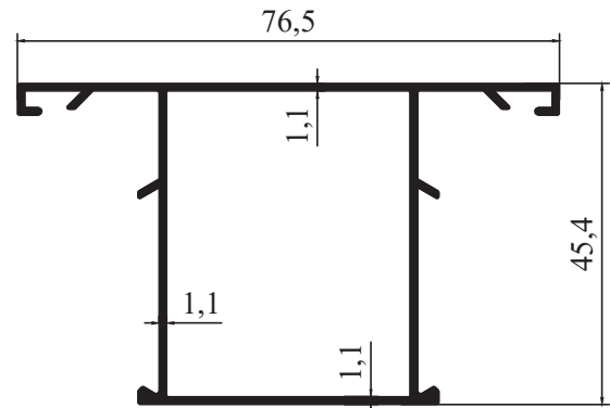
M 3006 - 0,706 kg/m
