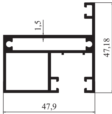
M 2054 - 0,962 kg/m
