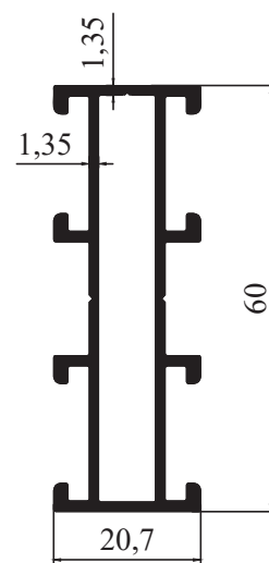
M 9515- 0,764 kg/m
