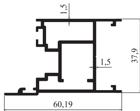
M 2157 - 0,954 kg/m
