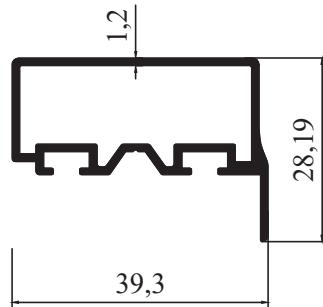
M 2154 - 0,463 kg/m
