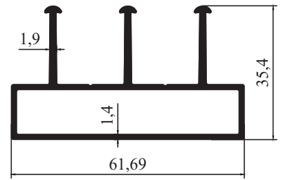
M 2212 - 0,900 kg/m
