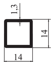
M 1416 - 0,151 kg/m
