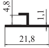
8900 - 0,094 kg/m
