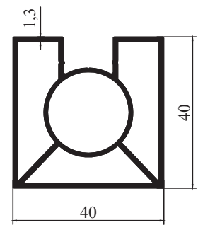
M 861 - 0,895 kg/m
