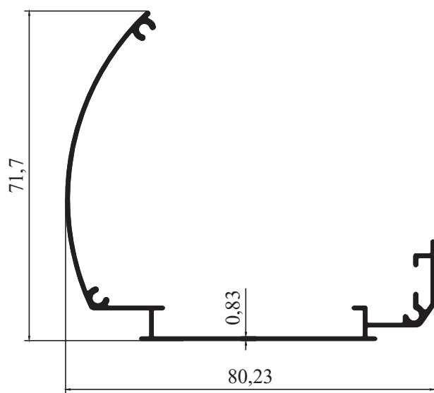
8000 - 0,480 kg/m
