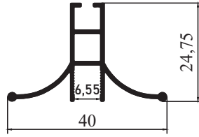
4145 - 0,284 kg/m
