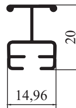
8877 - 0,168 kg/m
