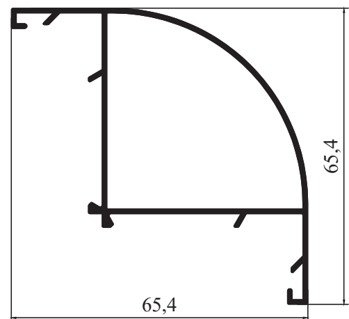
M 3011 - 0,703 kg/m
