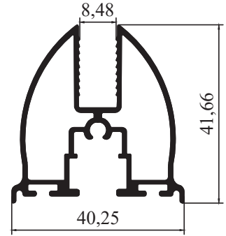
9125 - 0,705 kg/m
