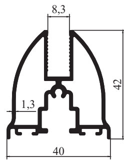
8444 - 0,816 kg/m
