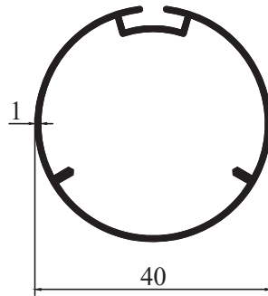
3119 - 0,390 kg/m
