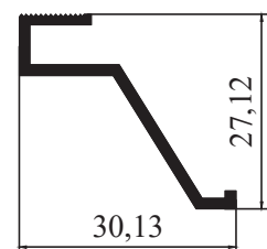
M 3022 - 0,227 kg/m
