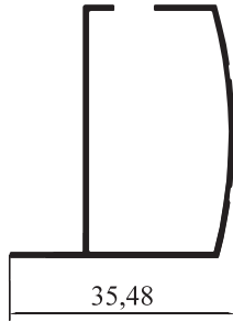
4468 - 0,333 kg/m STOK BOY : 5,80 cm
