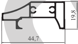
9246 - 0,498 kg/m
