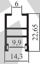
4465 - 0,244 kg/m
