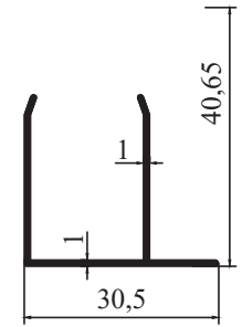
4453 - 0,222 kg/m STOK BOY : 5,80 cm
