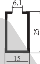
9120 - 0,276 kg/m STOK BOY : 6,00 cm
