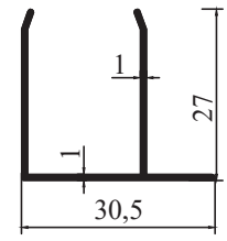
4453 - 0,222 kg/m STOK BOY : 5,80 cm
