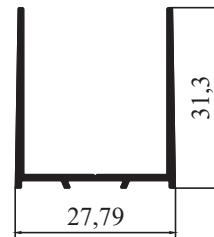
9089 - 0,292 kg/m STOK BOY : 6,00 cm
