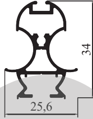
4251 - 0,430 kg/m STOK BOY : 5,40 cm
