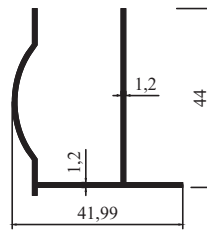
4421 - 0,410 kg/m STOK BOY : 6,00 cm
