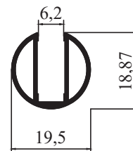
4377 - 0,236 kg/m STOK BOY : 6,00 cm
