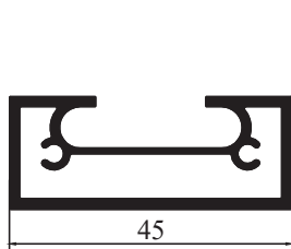
4467 - 0,658 kg/m
