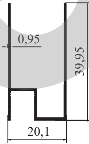
4118 - 0,273 kg/m
