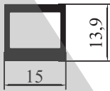
4459 - 0,268 kg/m
