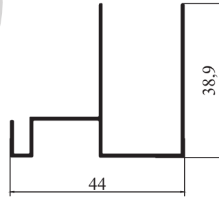
9248 - 0,336 kg/m
