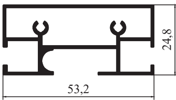
9088 - 0,685 kg/m STOK BOY : 6,00 cm
