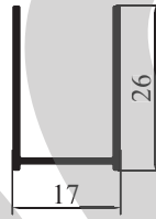
4466 - 0,206 kg/m
