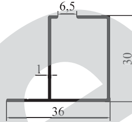
4144 - 0,289 kg/m STOK BOY : 5,80 cm
