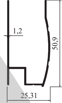
4122 - 0,413 kg/m STOK BOY : 5,80 cm
