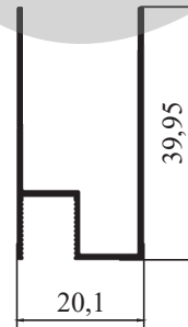
4118 - 0,273 kg/m
