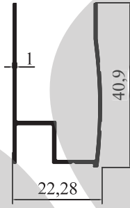
4123 - 0,302 kg/m STOK BOY : 5,80 cm
