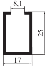
9121 - 0,285 kg/m STOK BOY : 6,00 cm
