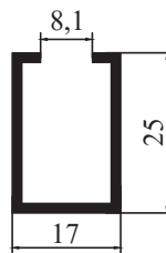
9121 - 0,285 kg/m STOK BOY : 6,00 cm
